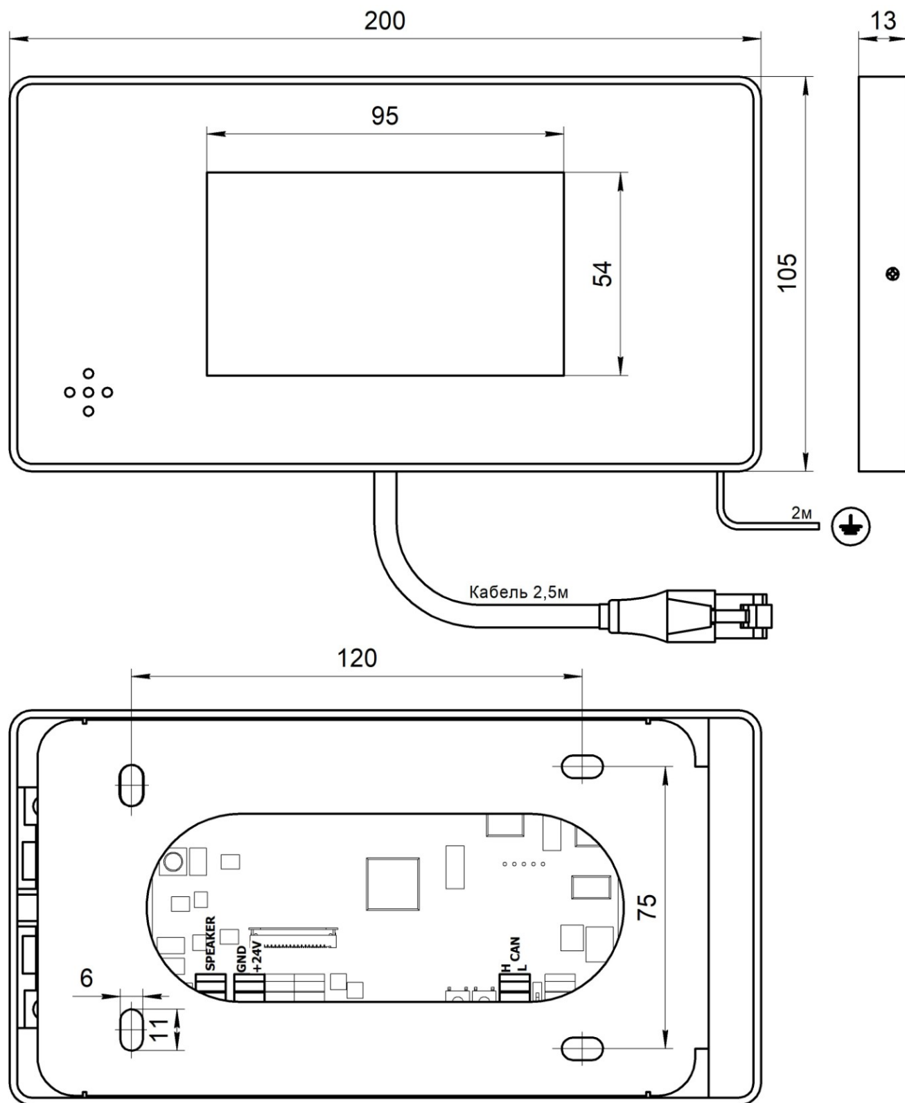
Рис.1 Внешний вид Табло накладное МАЛАХИТ (жгут RJ45) НШЕК.468232.132
